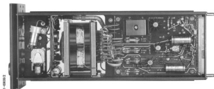
Bild 12. Batterie Stromversorgung BS 1500
