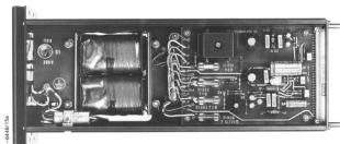
Bild 11. Netzstromversorgung NS 1500, Ansicht von rechts
