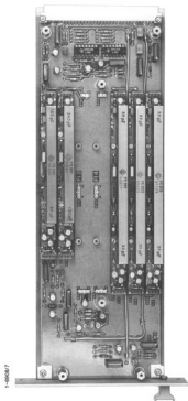
Bild 9. Filterbaugruppe FI 1510
