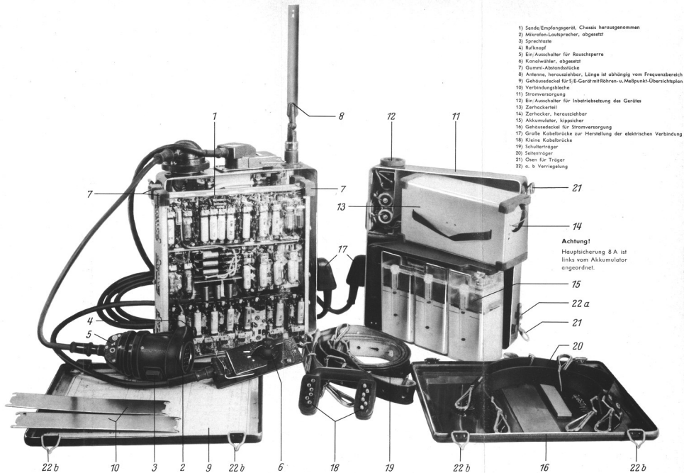
Abb. 8 Teleport IV. Bezeichnung der Einzelteile
