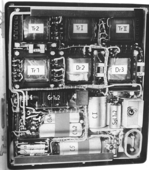
Abb. 24 Anordnung der Bauelemente der Teleport IV-Netz-Stromversorgung
