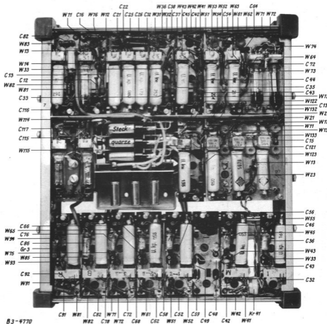
Abb. 23 Anordnung der Bauelemente des Teleport IV-Sende/Empfangsgerätes
