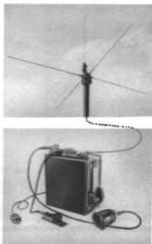
Abb. 18 S/E-Gerät mit Netz-Stromversorgung, Mikrophon-Lautsprecher und Antenne abgesetzt
