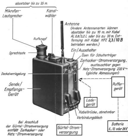
Abb. 9 Teleport IV, Anschlußmöglichkeiten für Zusatzgeräte
