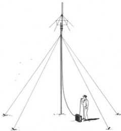
Abb. 4 Teleport IV mit Sende-Empfangs-Antenne für Schiffs- und Kurbelmaste
