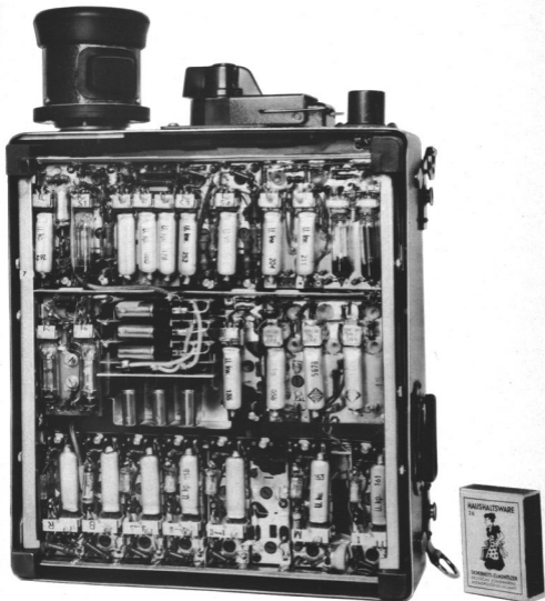
Abb. 2 Teleport IV, Innenansicht des Sende/Empfangsteiles Oberes Drittel: Senderteil Mittleres Drittel: NF-Verstärker, Steckquarze und Empfänger-Eingangsteil Unteres Drittel: ZF-Verstärker und Rauschperre
