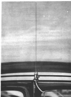
Abb. 22 Autoantenne am Regenablauf eines Volkswagens montiert
